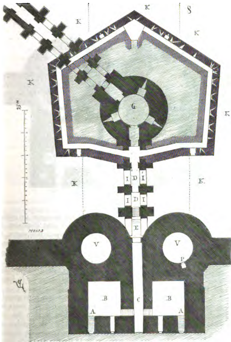
La figure 9 donne le plan de la porte, au niveau du pavé de la ville. Ce plan montre le passage pour les chariots et les piétons, se rétrécissant vers l'entrée extérieure.
